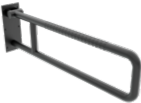
Novinka Sklopné podpěrné madlo 800 mm Tvaru U. Průměr 32 mm. Povrch barva černá matná. Nerezová ocel 18/8.
