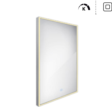
LED zrcadlo 500 x 700 S dotykovým senzorem. Možnost nastavení teploty svítivosti od 2700K - 6000K. Výkon 35W. Rám hliníkový.
