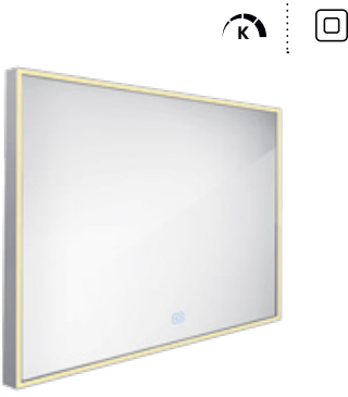
LED zrcadlo 900 x 700 S dotykovým senzorem. Možnost nastavení teploty svítivosti od 2700K - 6000K. Výkon 47W. Rám hliníkový.
